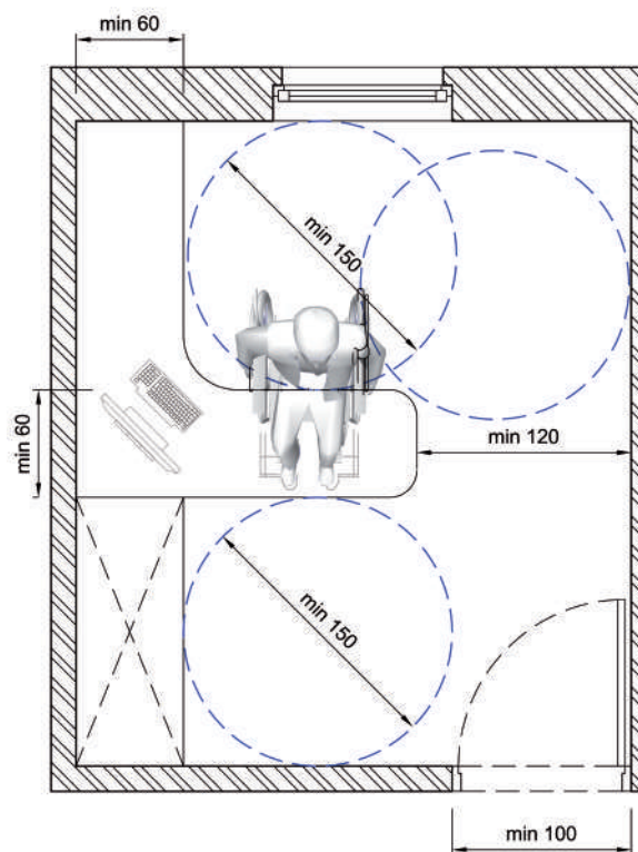
Inrichtingsvoorbeeld van een individueel kantoor
