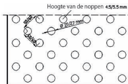
✓ Roestvast stalen plaat, in te gieten
